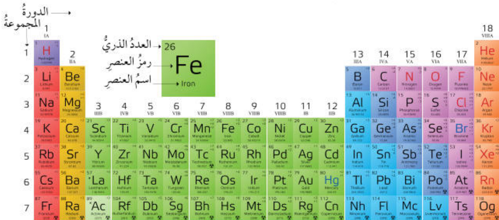
الشكل (16): الجدول الدوري الحديث للعناصر.
