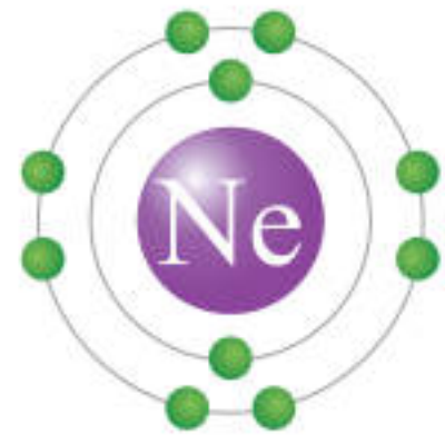
الشكل (33): توزيع ذرة النيون المستقرة.
