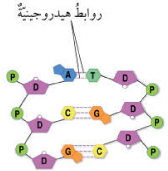
الشكل (4): ارتباط القواعد النيتروجينية في جزيء DNA.
