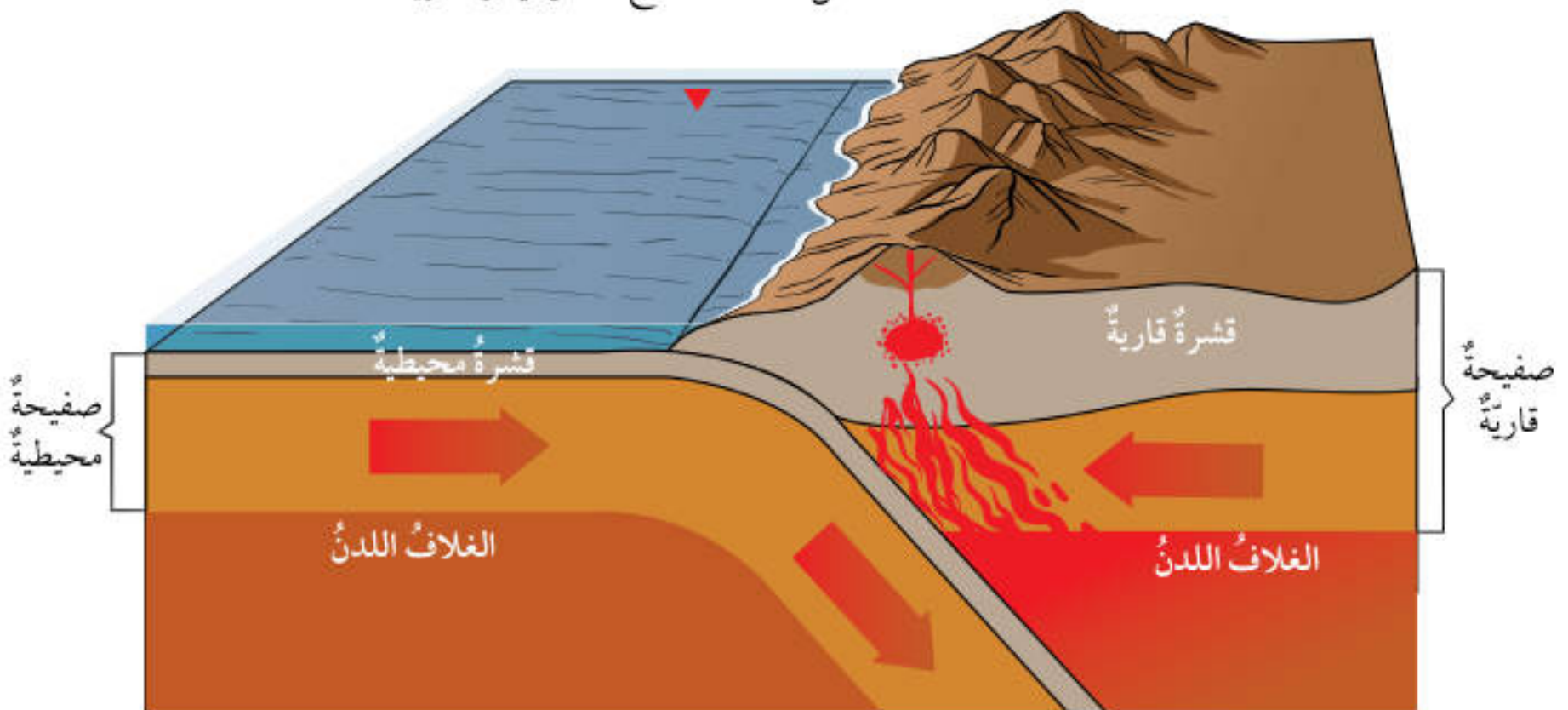
الشكل (2): الصفائحُ المحيطيةُ والقاريةُ.
