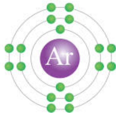
الشكل (34): توزيع ذرة الأرجون المستقرة.
