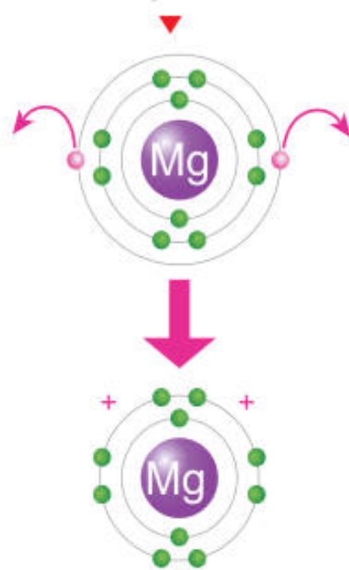
الشكل (36): تكوين أيون المغنيسيوم \text{Mg}^{2+} .
