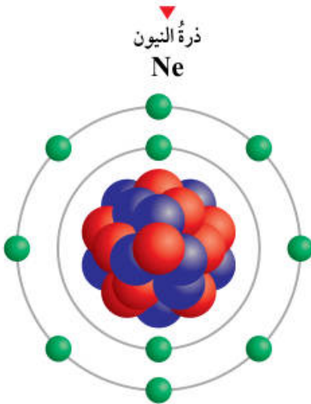
الشكل (24): توزيع ذرة عنصر النيون.
