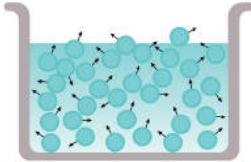
الشكل (5): ضغط السائل يؤثر في جدران الوعاء الذي يحويه وقاعدته.
