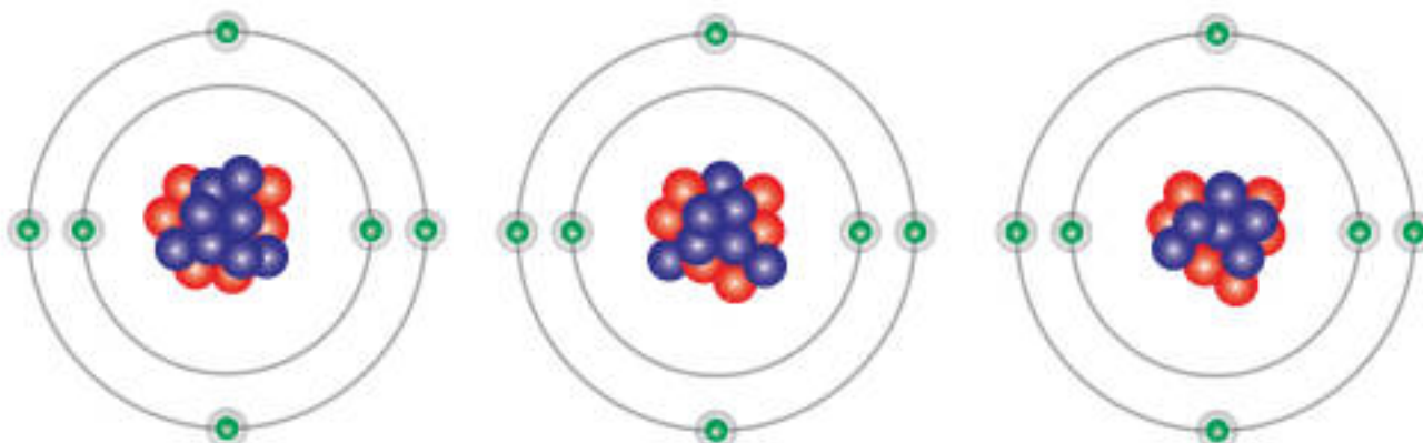
نواة C-14 ^{14}_6\text{C}
