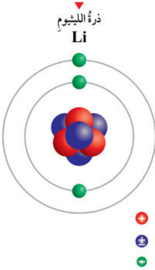
الشكل (22): توزيع ذرة عنصر الليثيوم.
