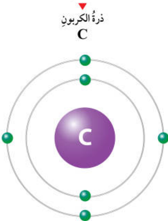
الشكل (30): توزيع ذرة عنصر الكربون.
