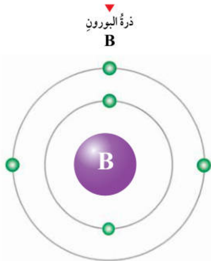
الشكل (29): توزيع ذرة عنصر البورون.
