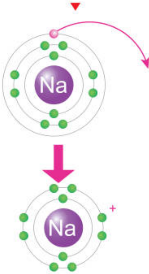
الشكل (35): تكوين أيون الصوديوم \text{Na}^+ .
