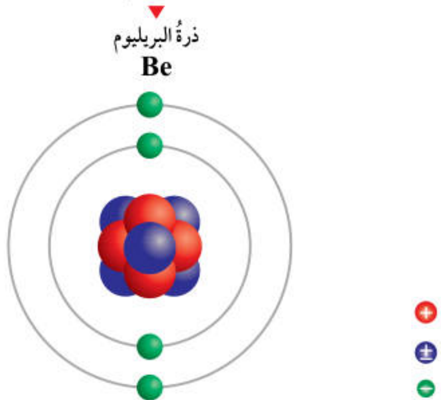
الشكل (23): توزيع ذرة عنصر البريليوم.
