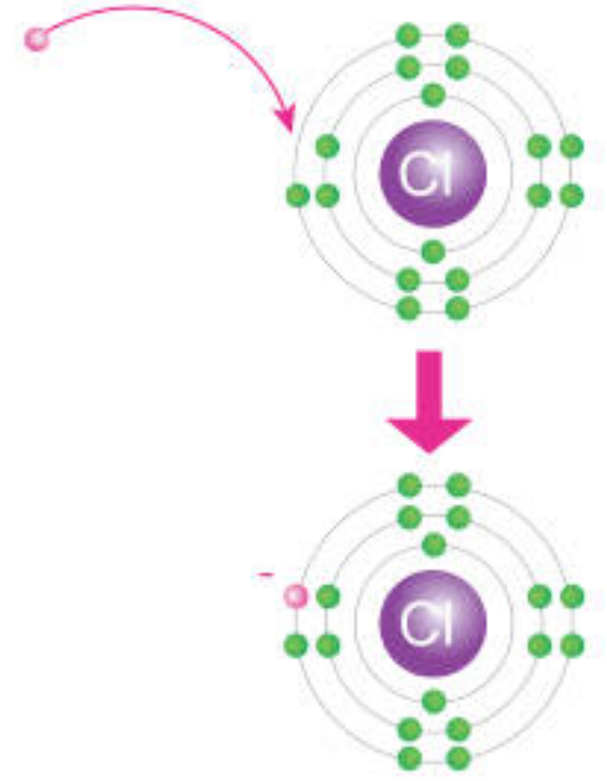
الشكل (37): تكوّن أيون الكلوريد \text{Cl}^- .
