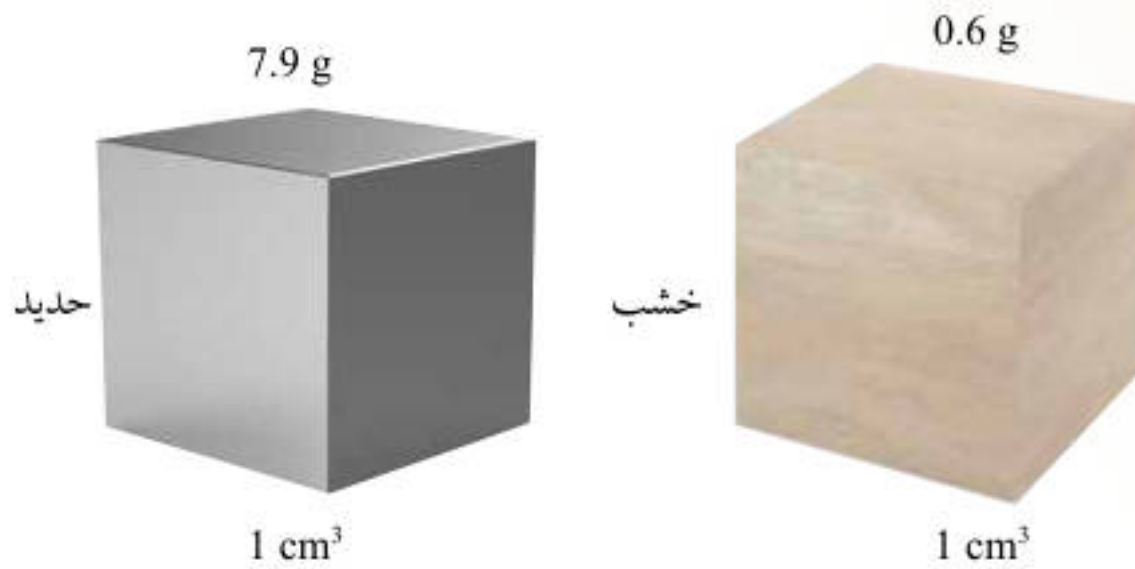
الشكل (13): تختلف الكثافة باختلاف نوع المادة.
