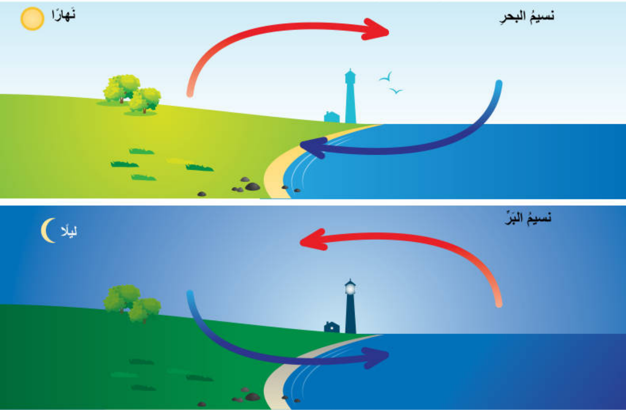
الشكل (6): آلية حدوثِ نسيمِ البرِّ ونسيمِ البحرِ.
