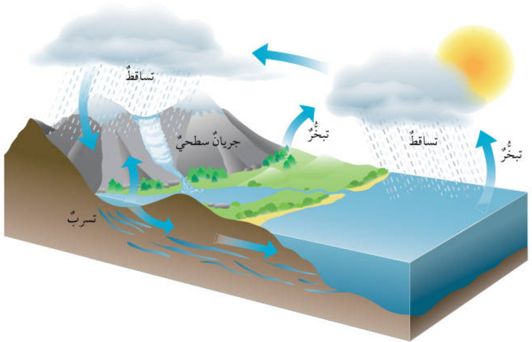
الشكل (7): دورة المياه في الطبيعة.
