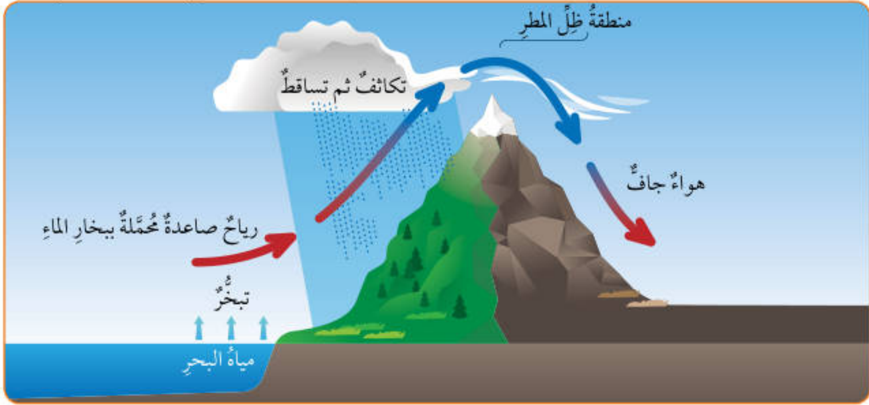
الشكل (8): كيفية حدوث الأمطار التضاريسية.
