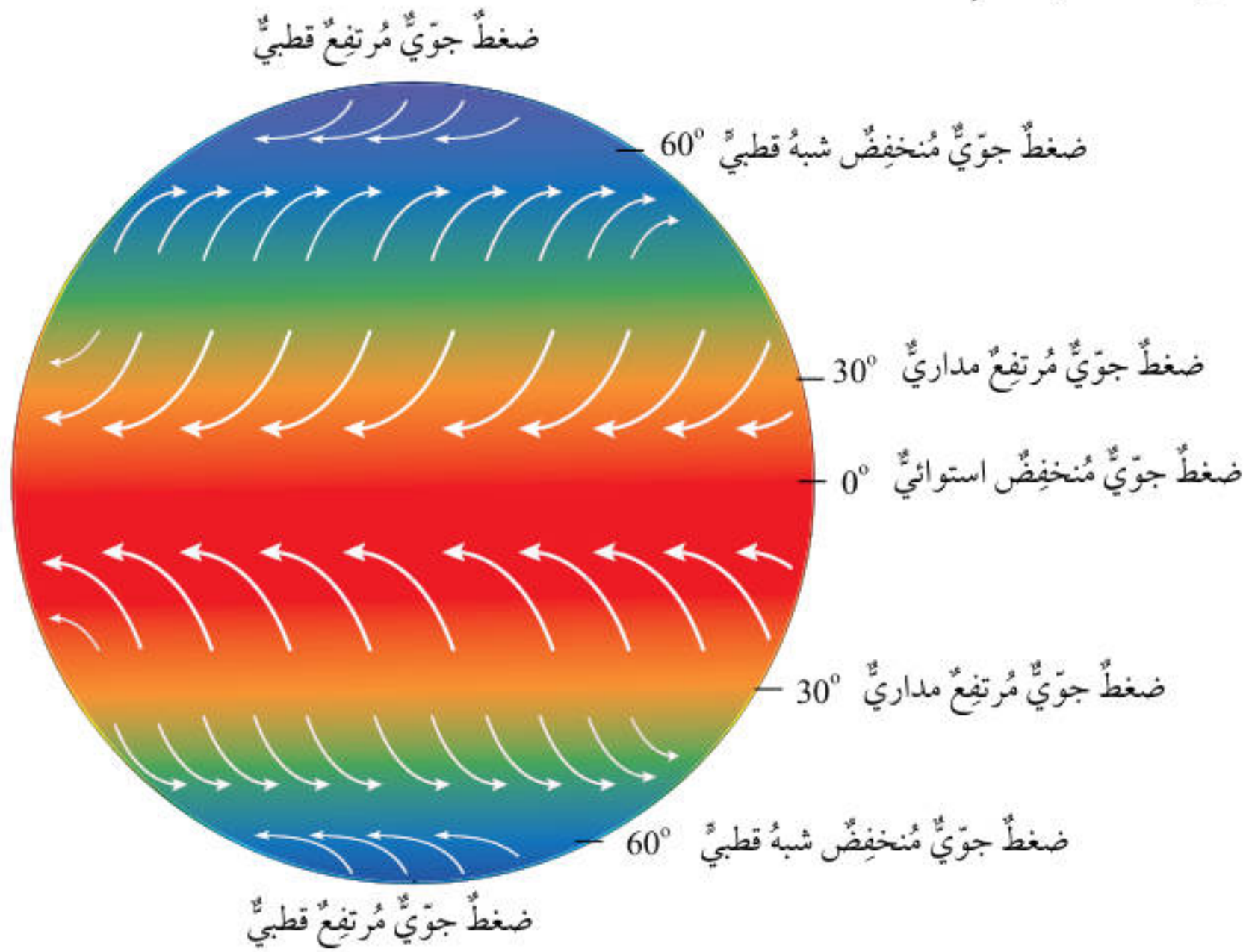
الشكلُ (3): نطاقاتُ الضغطِ الجوّيِّ الرئيسيّةِ في العالمِ.
