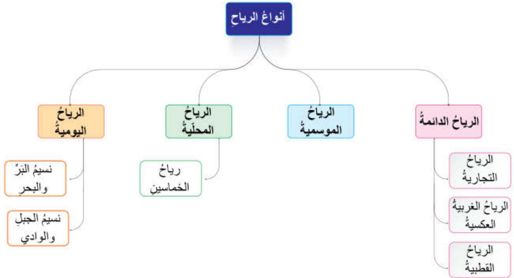
الشكل (5): أنواع الرياح.
