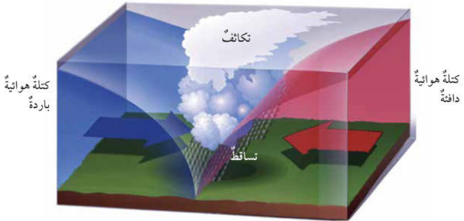
الشكل (10): كيفية حدوث الأمطار الإعصارية.
