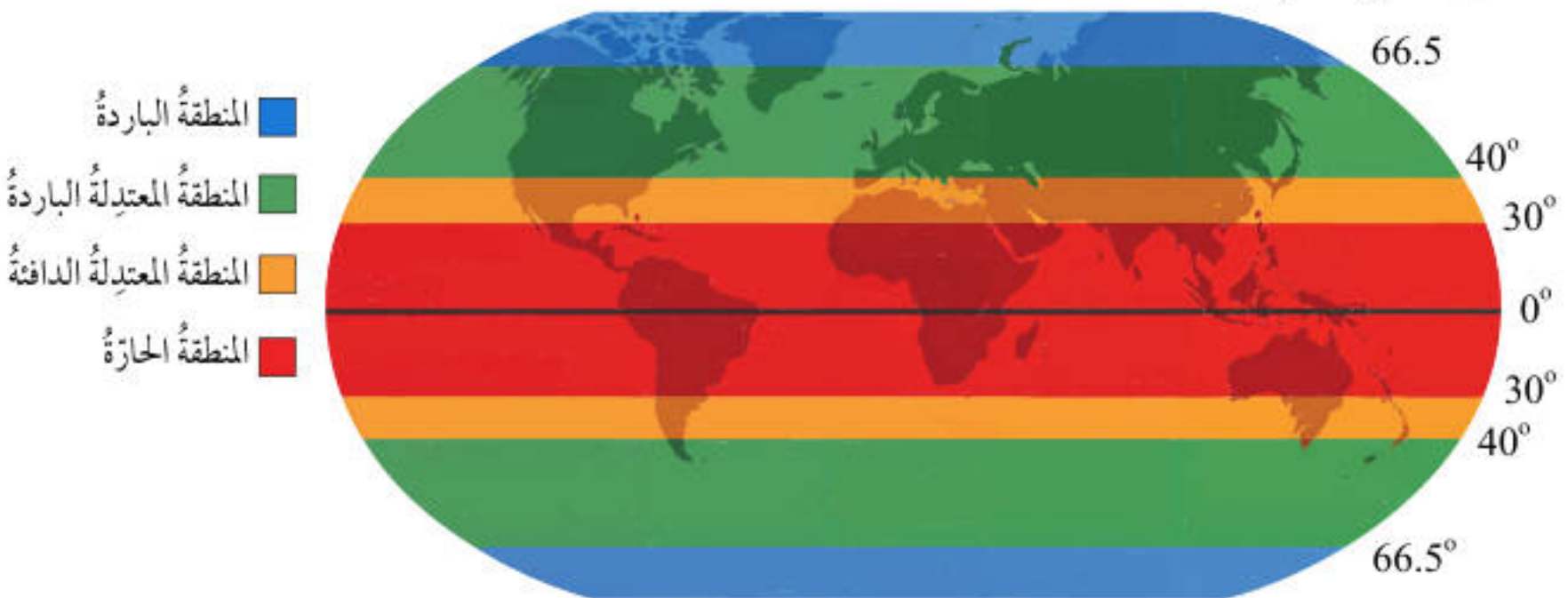
الشكل (1): المناطق الحرارية الرئيسية في العالم.
