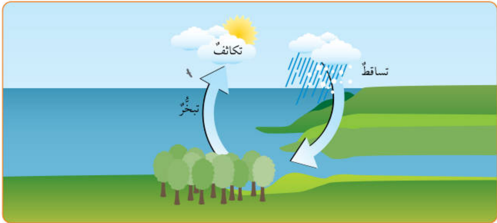
الشكل (9): كيفية حدوث الأمطار الحملية.
