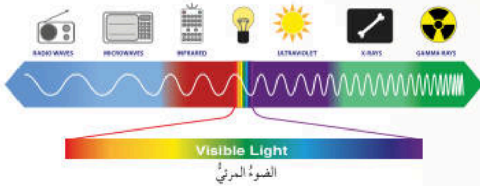
الشكل (1): أقسام الموجات الكهرومغناطيسية.
