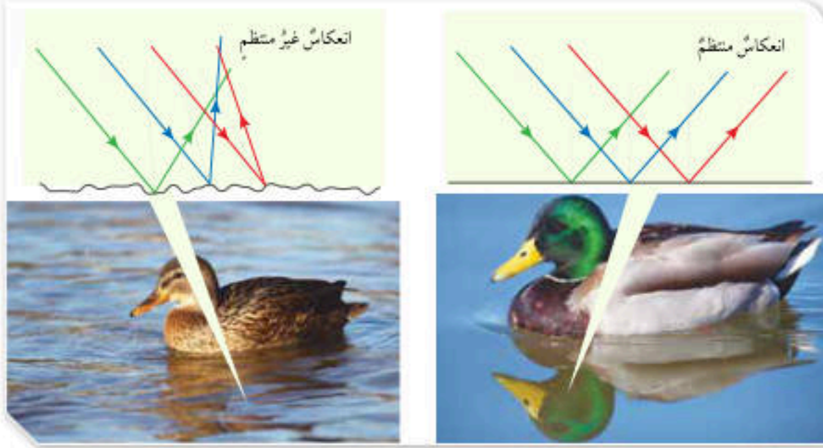
الشكل (3): انعكاس الضوء منتظم وغير منتظم.
