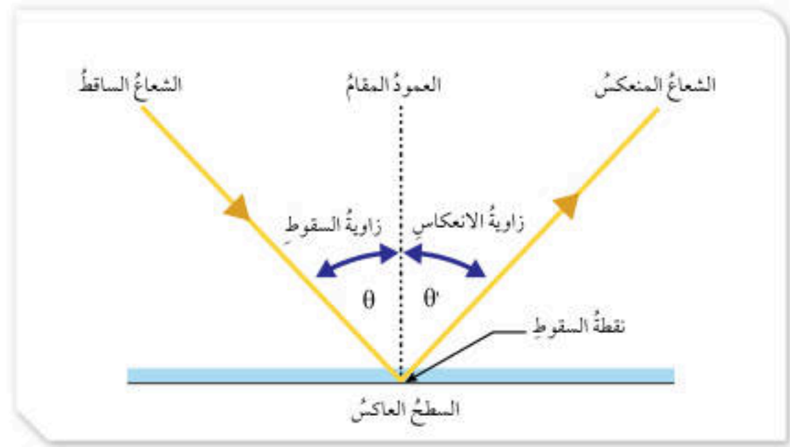
الشكل (4): زاوية السقوط والانعكاس.
