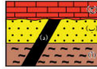
الشكل (7): تعاقبات لصخور رسوبية (أ، ب، ج)، وقاطع صخري ناري (د).
