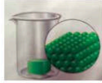
الشكل (2): ترتيب جسيمات المادة في الحالة الصلبة.
