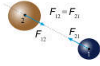
الشكل (15): القوى في الطبيعة دائماً على شكل أزواج.
