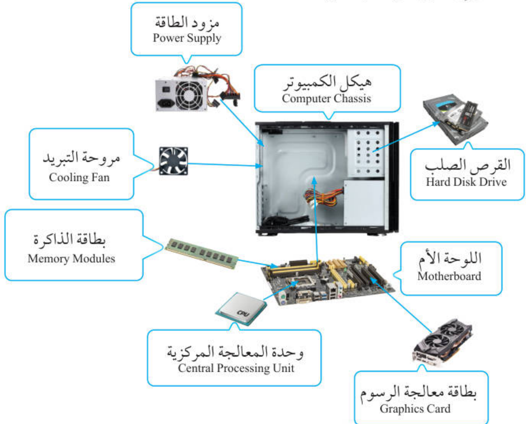
الشكل (2-2): أهم الأجزاء الداخلية لجهاز الحاسوب.
